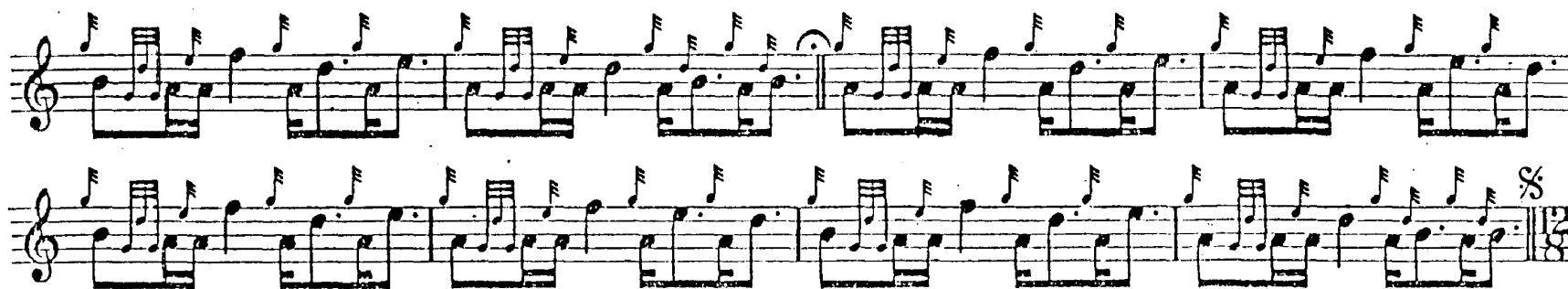
Ex: Taor-luath.*
